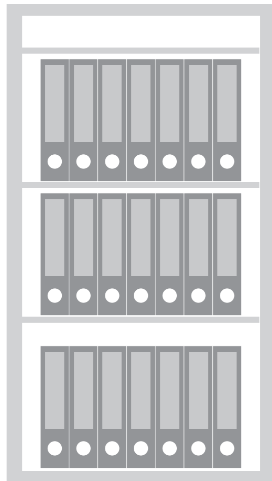
Modell Potsdam 37100 Außenmaß 1250 x 700 x 500 mm Innenmaß 1190 x 630 x 375 mm
